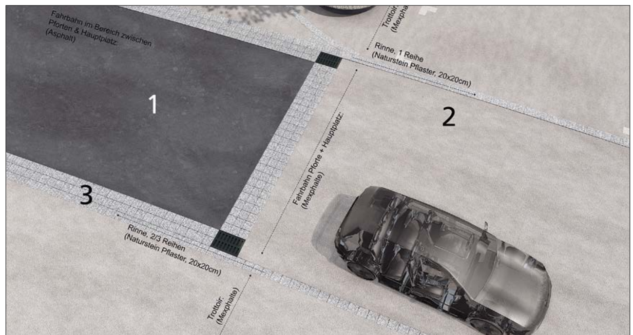
Materialisierung von Fahrbahn, Gehbereichen und Randabschlüssen: Asphalt (1), «Mexphalt» (2) und Natursteinpflaster (3).
