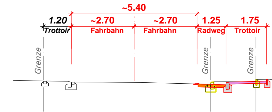
Querprofil 5, 1:100
