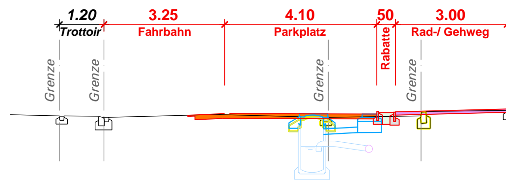
Querprofil 4, 1:100
