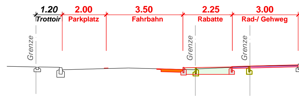
Querprofil 4, 1:100
