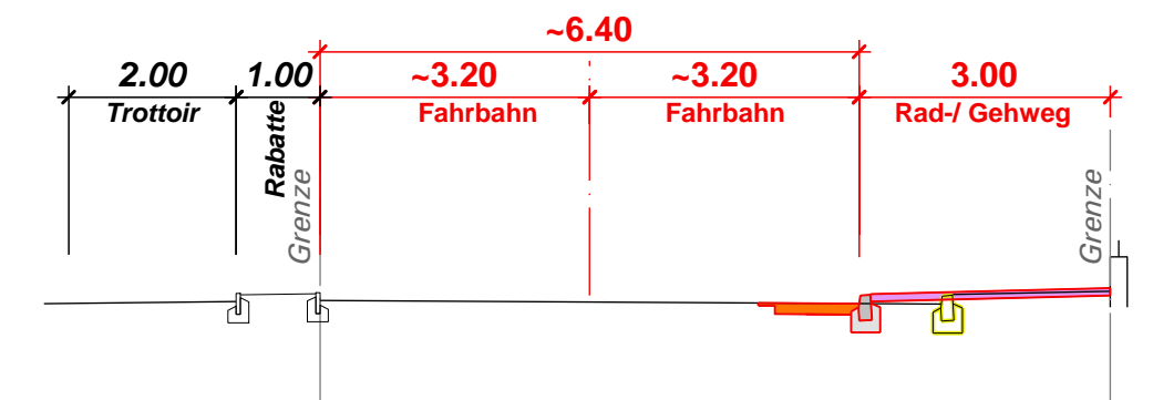
Querprofil 6, 1:100
