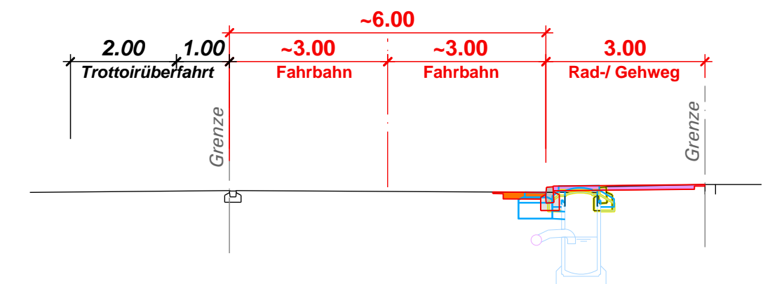
Querprofil 7, 1:100
