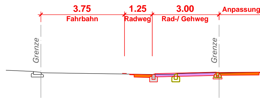
Querprofil 3, 1:100
