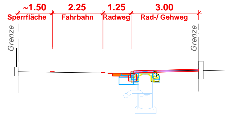
Querprofil 2, 1:100
